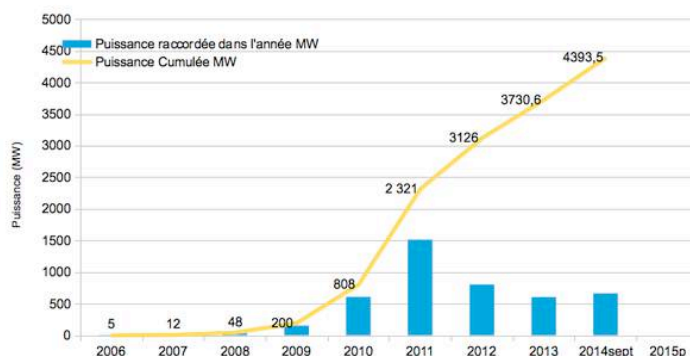
Parc photovoltaïque français raccordé au réseau géré par ERDF
